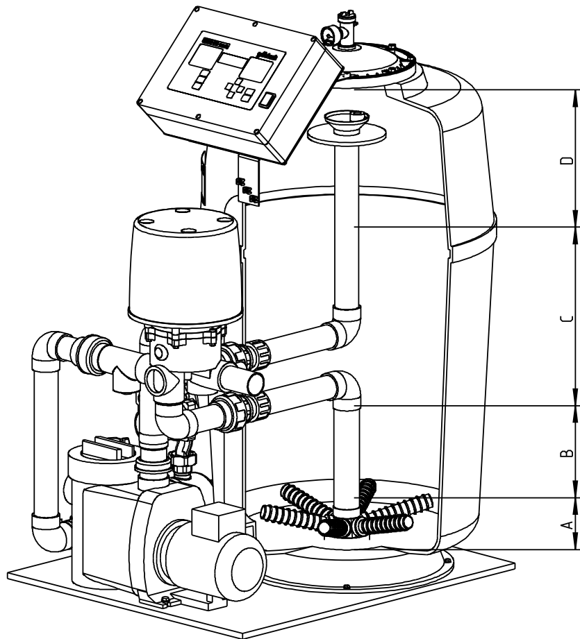
Abb. C-5: Schüttschema zu GENO-mat® F 600 AK
