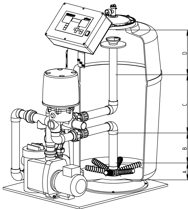
Abb. D-2: Schüttschema zum GENO-mat® F 600 AK
