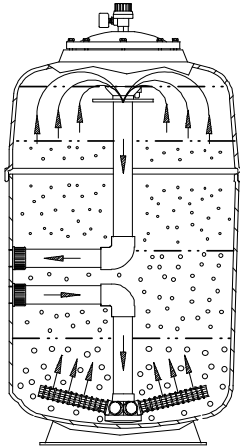
Abb. B-3: Rückspülen GENO-mat® 600
